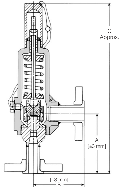
Flange x Flange
